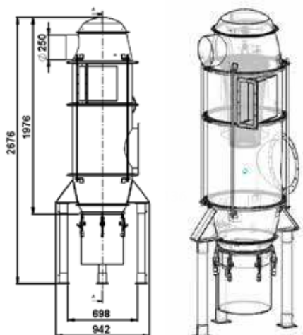
S 21000 EX
