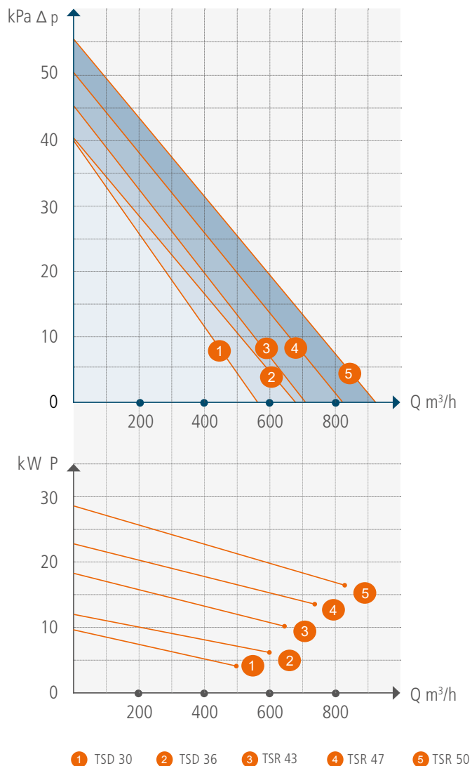
Turbopumps TSD/TSR
